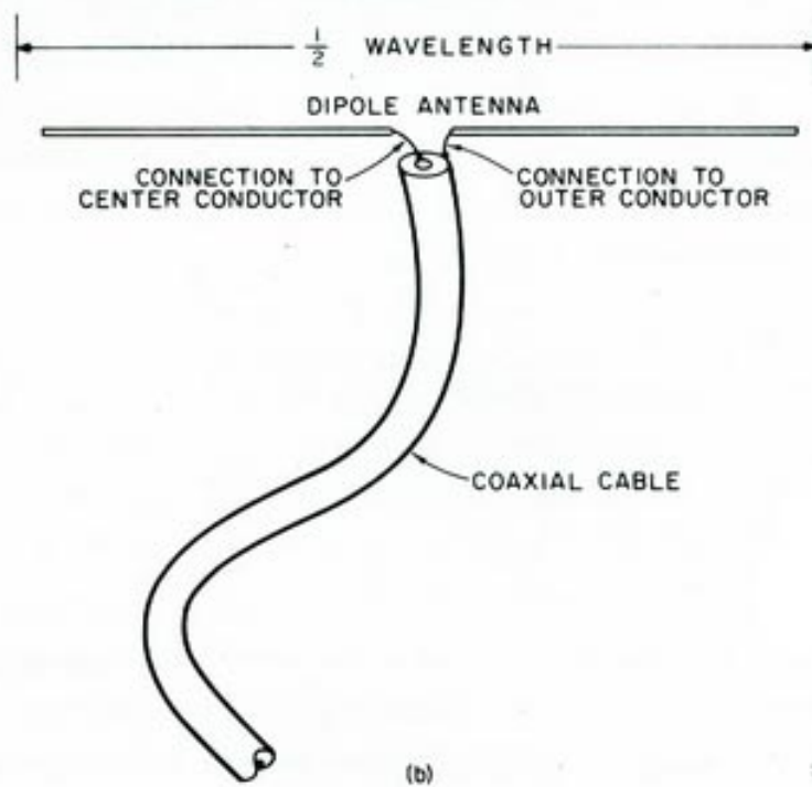
FIG. 5 DIPOLE ANTENNA
